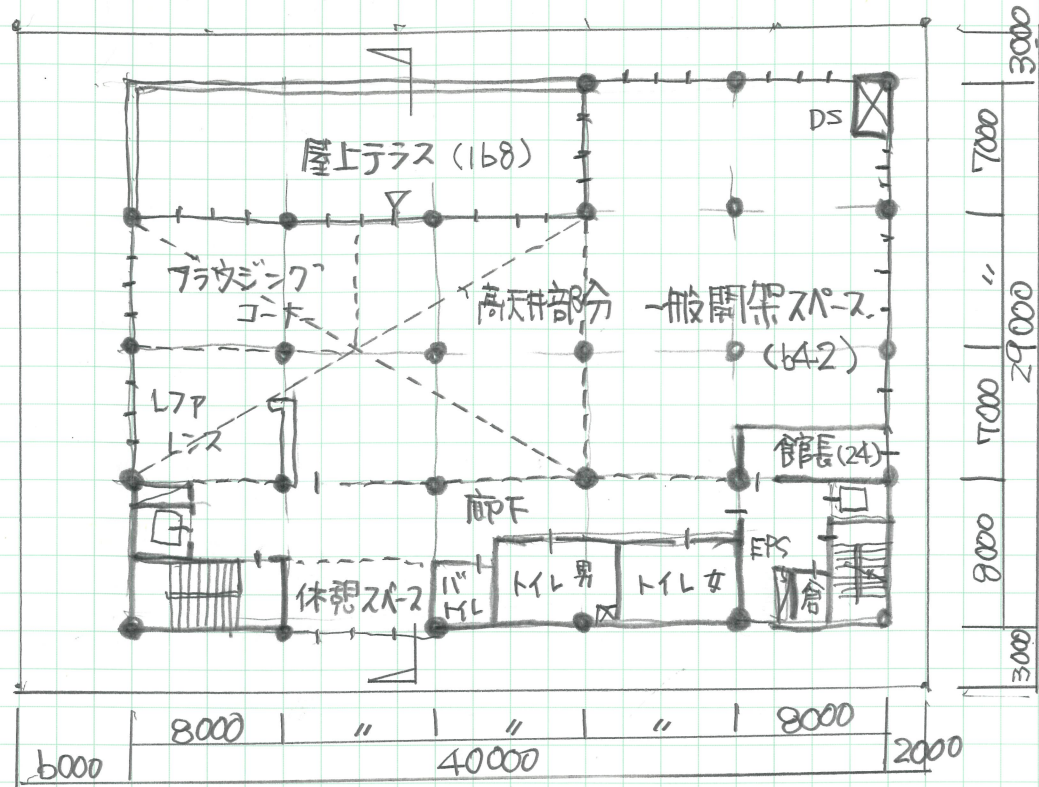
3階平面図 1/400
