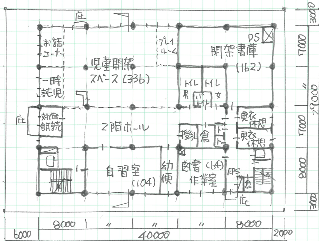
2階平面図 1/400
