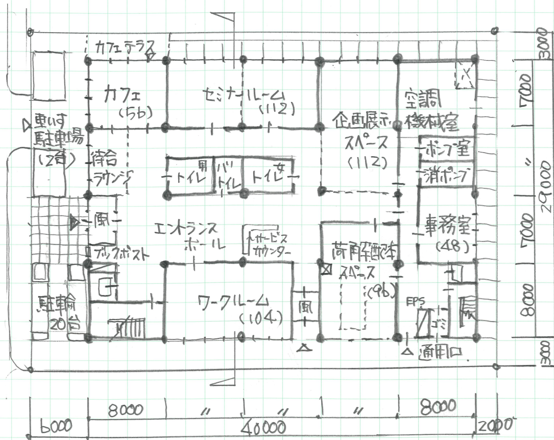
1階平面図, 配置図 1/400
