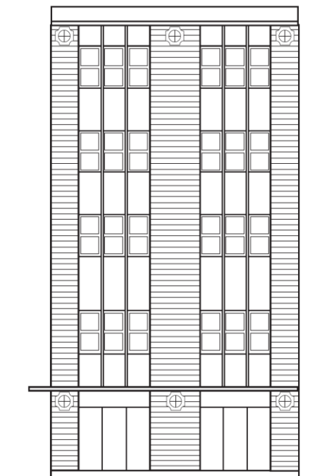
南側立面图
