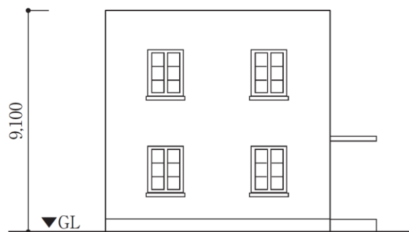
南側立面图
