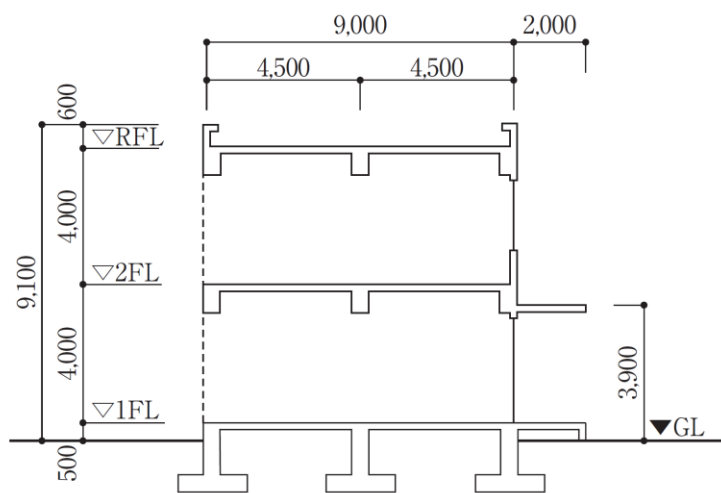
A - A' 断面图
