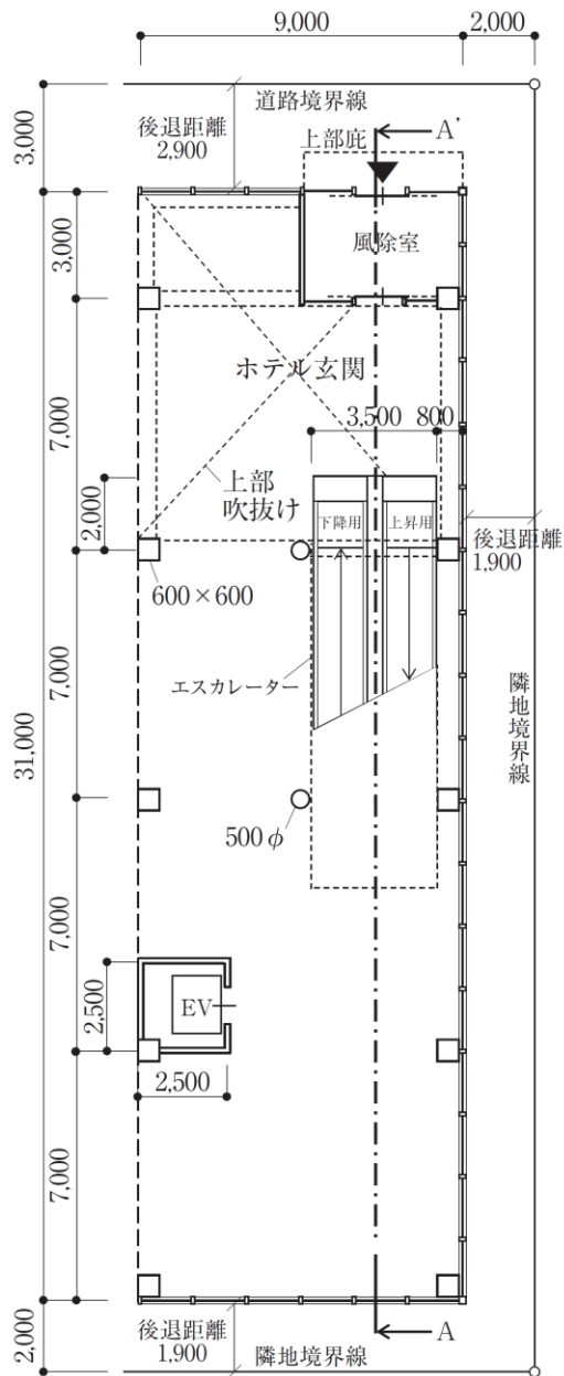
1階平面図
