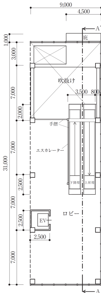
2階平面図
