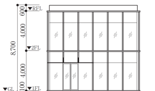
北側立面図
