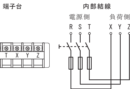
図3. 開閉器代用の端子台説明図
