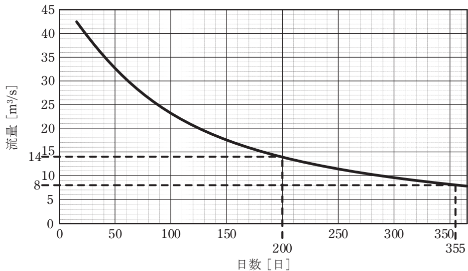
図 流況曲線
